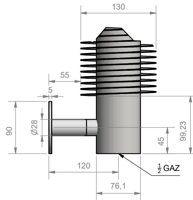
Détail A ( 0.5 : 2 )
